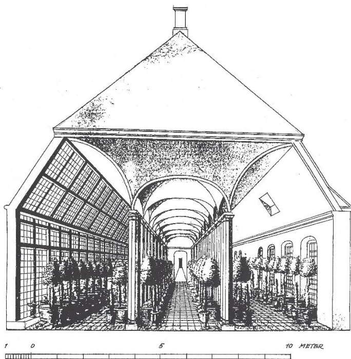
Fig. 86. Tværsnit af orangeriet ved Fredensborg Slot med datidens nye mansardtag gengivet af H. C. Lønborg 1728. (SCC foto, 1997).
