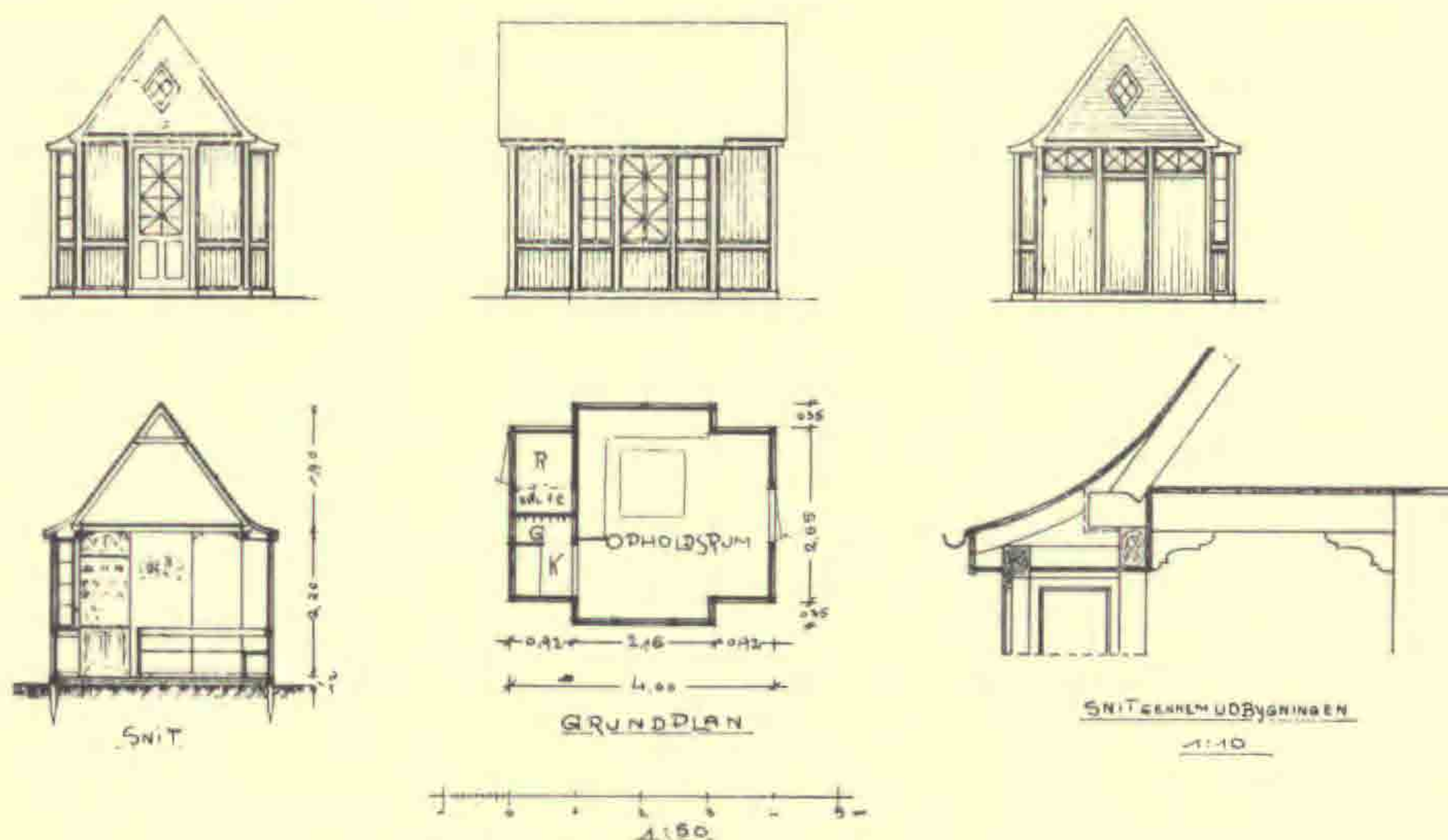
Tegning til et pænt, lille Kolonihavehus.
